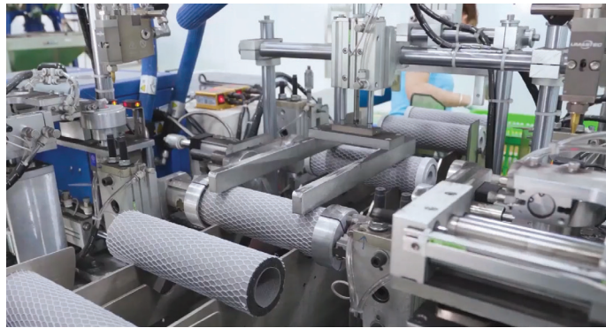
Dây chuyền sản xuất lõi lọc nước
